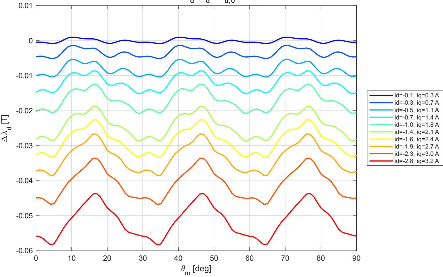
Differenza Assoluta \lambda_d ( \lambda_d - \lambda_{d,0} ) lungo MTPA
