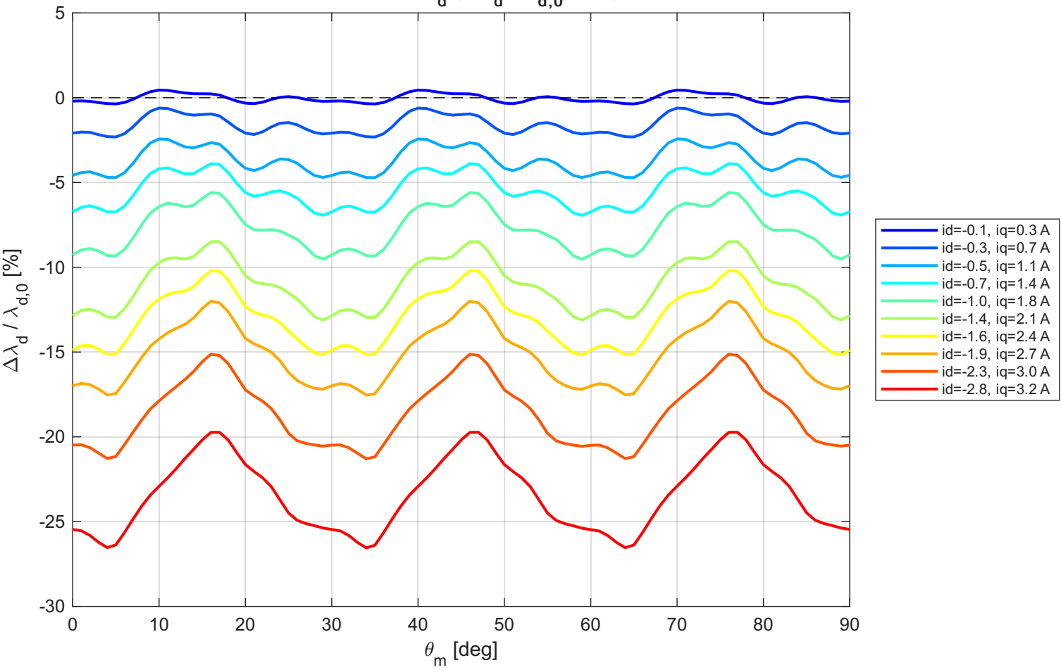
Variazione Relativa \lambda_d ( \Delta\lambda_d / \lambda_{d,0} ) lungo MTPA
