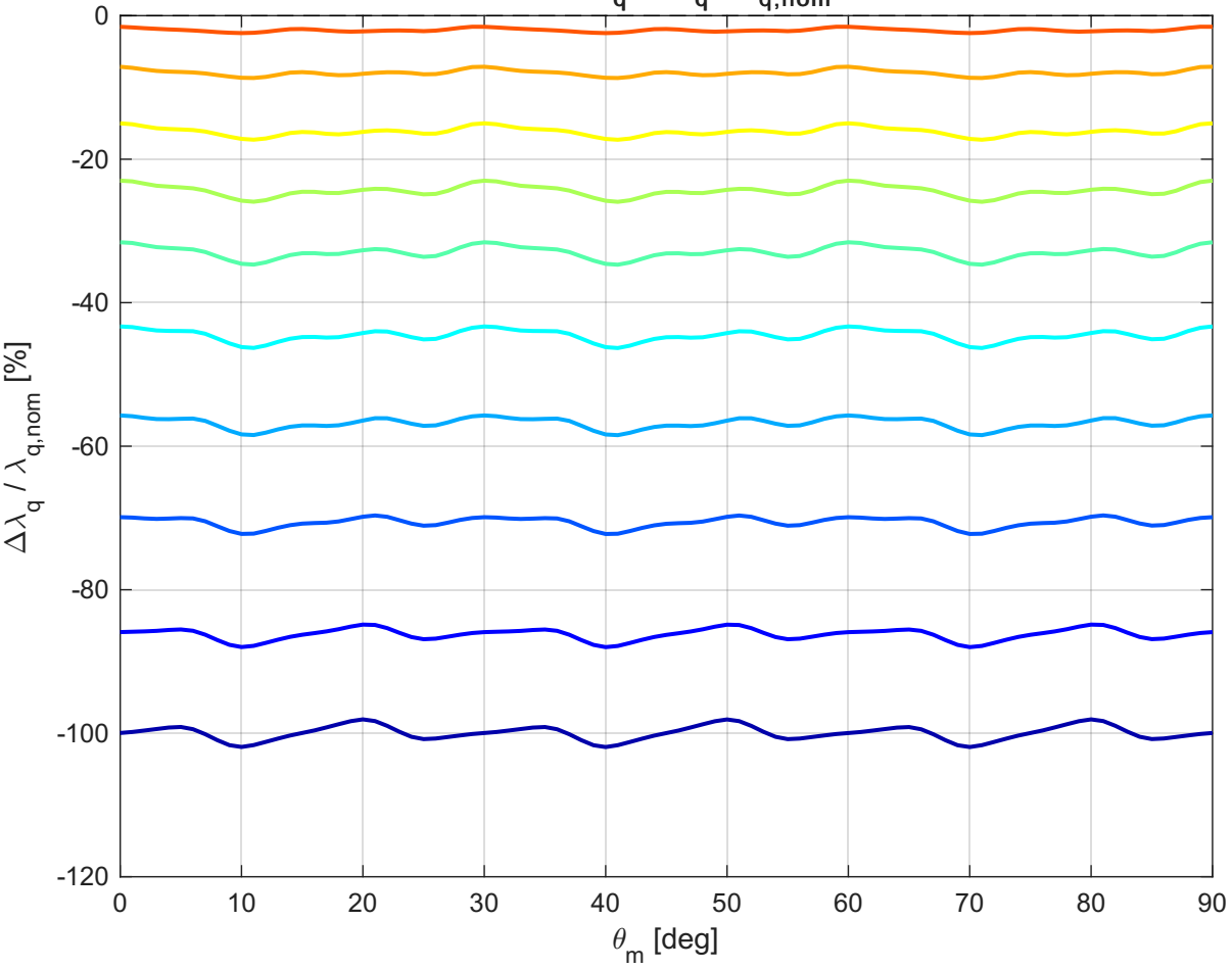
Variazione Relativa \lambda_q ( \Delta\lambda_q / \lambda_{q,nom} ) lungo MTPA
