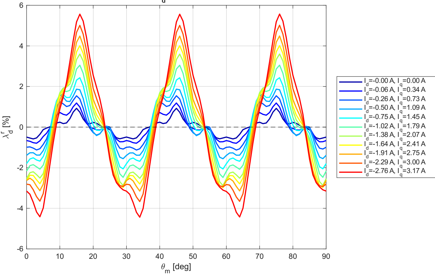
Ripple Relativo di \lambda_d lungo la traiettoria MTPA
