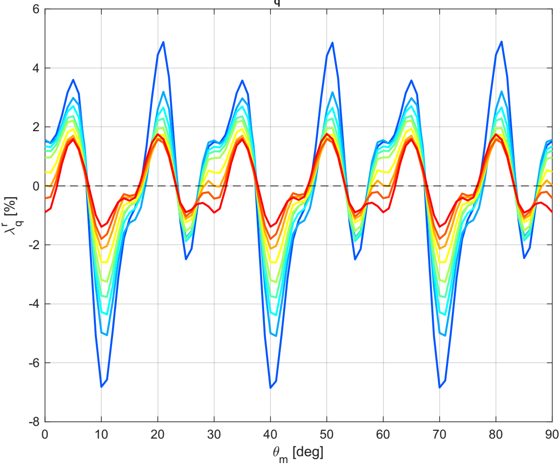
Ripple Relative di \lambda_q lungo la traiettoria MTPA
