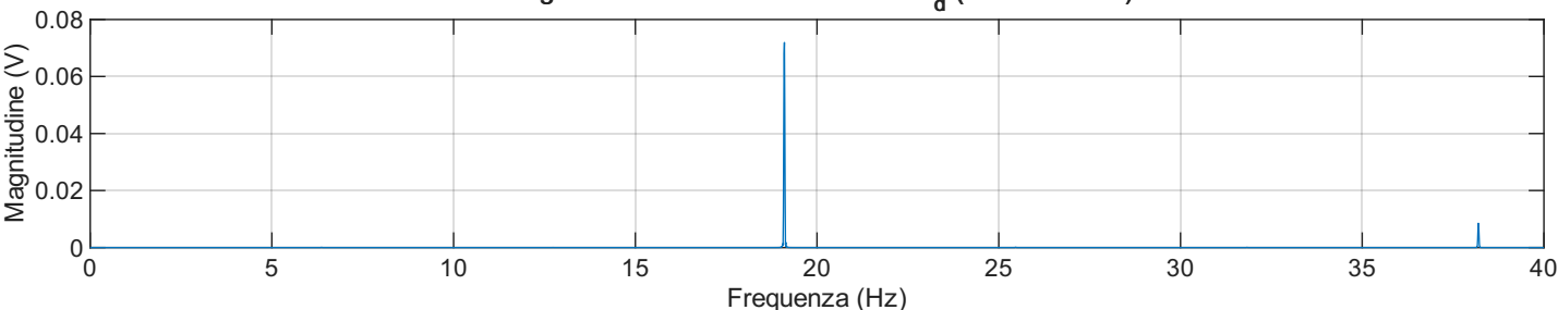
Magnitudine FFT del disturbo di e_d ( \omega = 100 rad/s)
