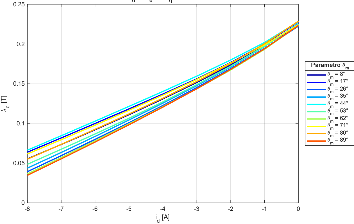
\lambda_d vs i_d (@ i_q = -1 A)
