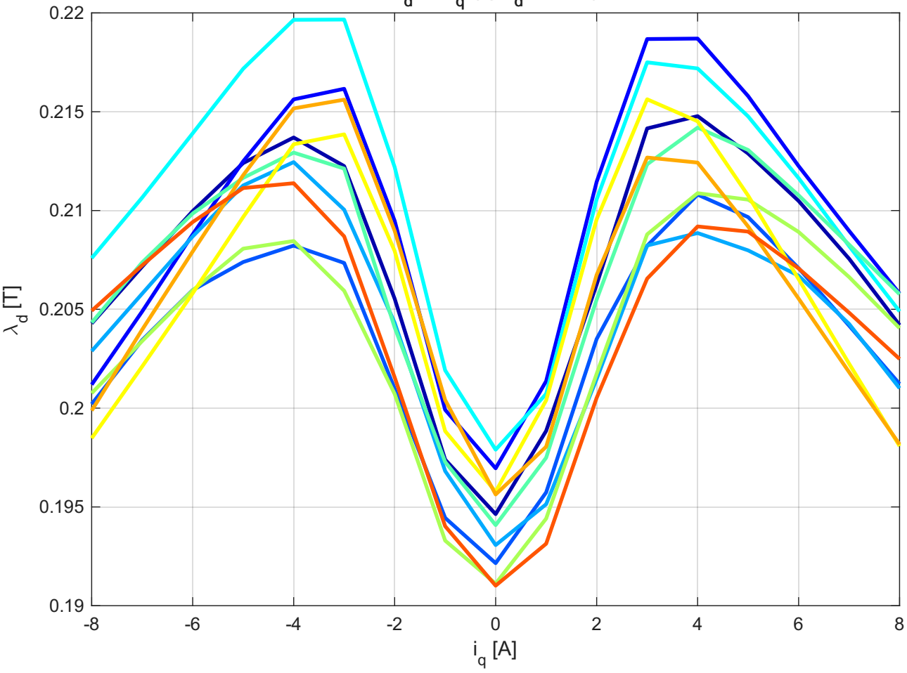
\lambda_d vs i_q (@ i_d = -1 A)
