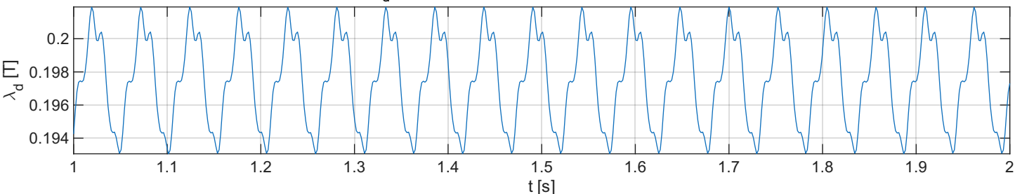
\lambda_d (velocità 100 rad/s; id = -1 A, iq = -1 A)
