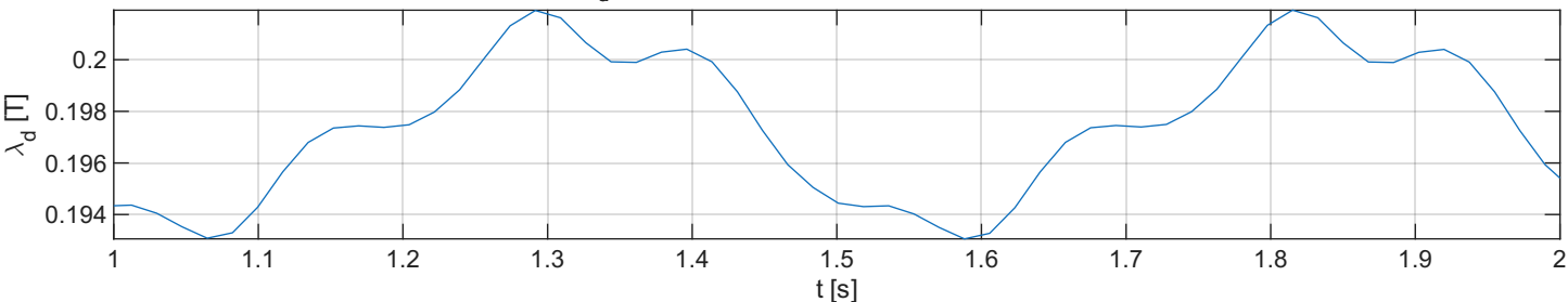
\lambda_d (velocità 10 rad/s; id = -1 A, iq = -1 A)
