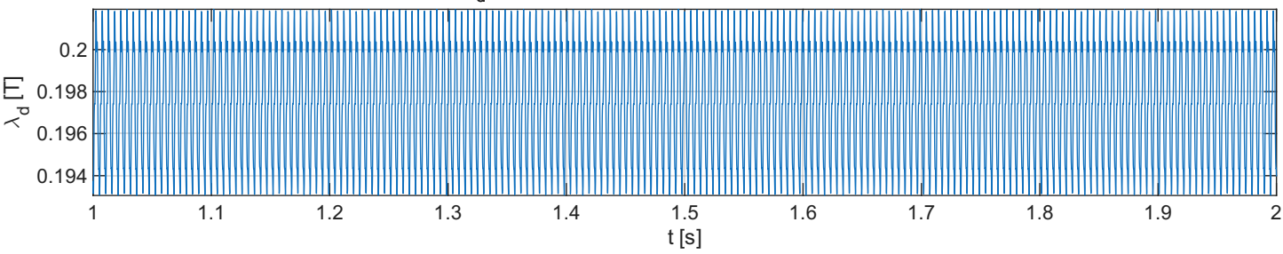
\lambda_d (velocità 100 rad/s; id = -1 A, iq = -1 A)
