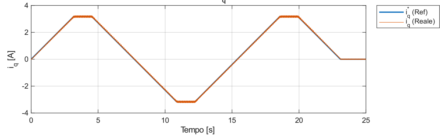
Andamento i_q
