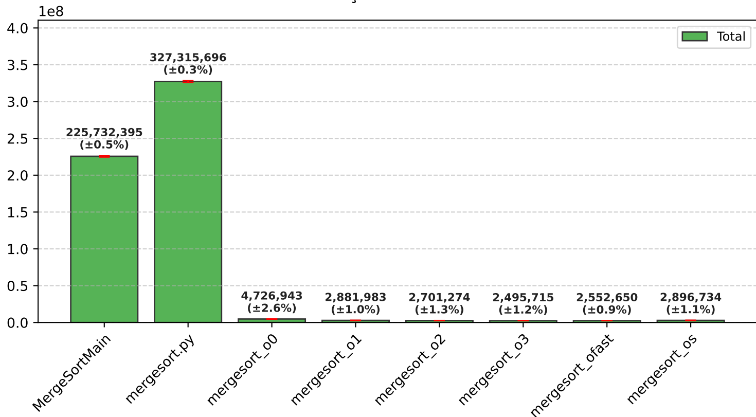
Page Faults
