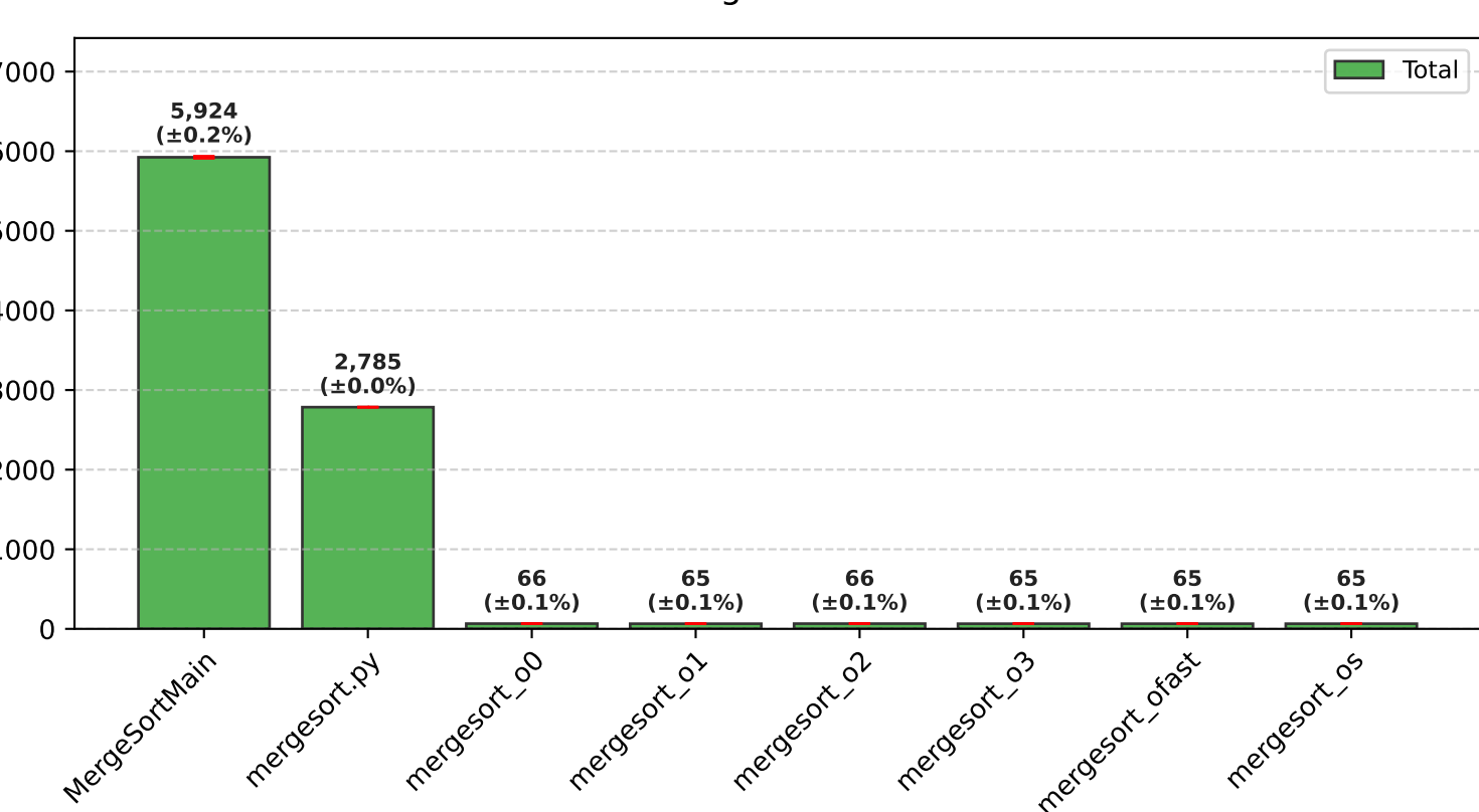
Page Faults
