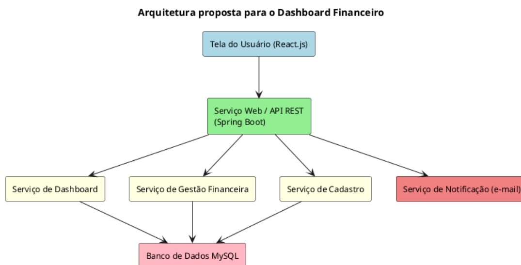
Figura 3.1 – Arquitetura proposta para o Dashboard Financeiro .
