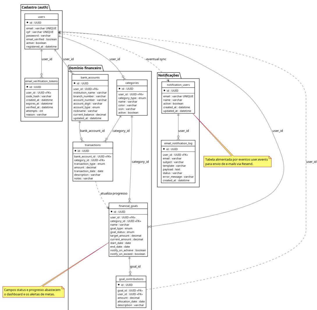
Figura 3.2 – Modelo relacional consolidado no MySQL.
