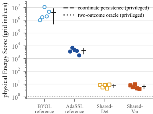
(b) MPI3D
