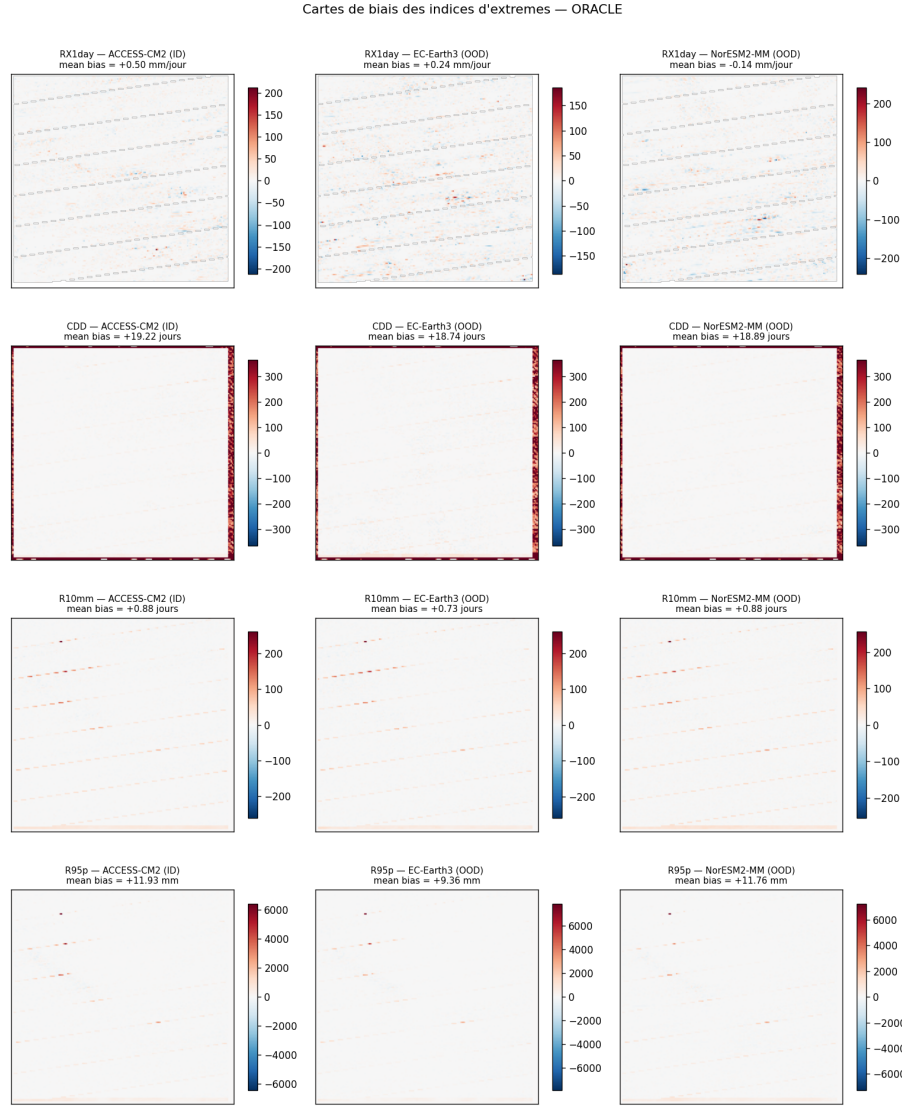
Figure 14 — Biais sur l'indice RX1day pour ORACLE. Le déficit, concentré sur le versant occidental des Southern Alps , révèle l'absence d'orographie HR (DEM) en entrée. Le même schéma spatial s'observe sur CORRDIFF , ce qui montre que la cause est l'information manquante, pas la causalisation.
