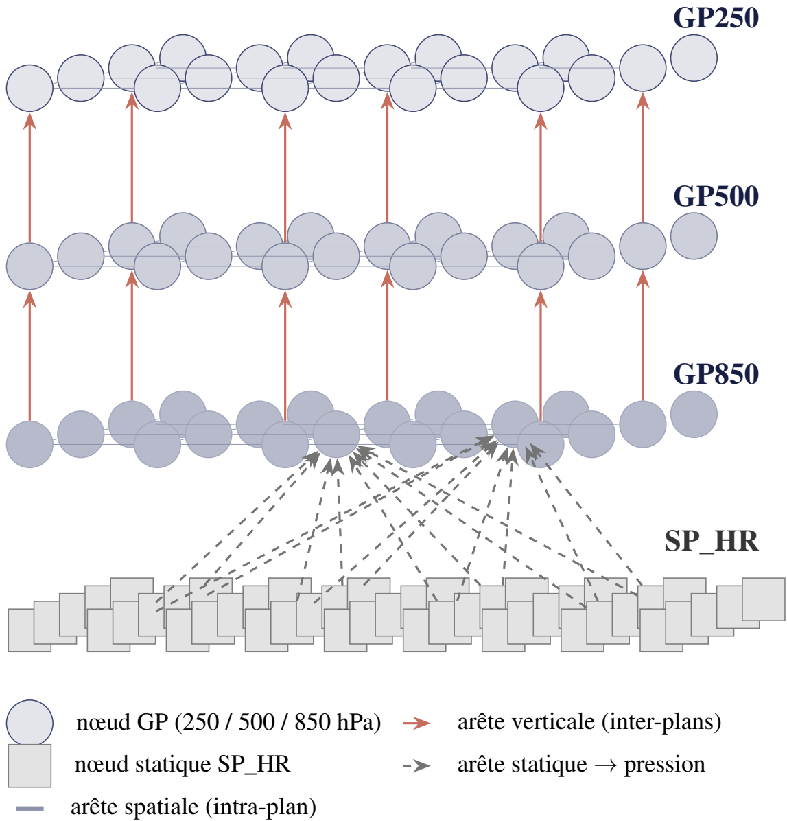
FIGURE 8 – Vue conceptuelle du graphe atmosphérique hétérogène d’ORACLE. Quatre types de nœuds (GP850, GP500, GP250 dynamiques en bleu; SP_HR statique en gris) et trois types d’arêtes (spatiales intra-plan en bleu clair, verticales inter-plans en rouge, statiques-vers-pression en pointillé gris). L’instanciation concrète avec variables nommées et dimensions exactes est différée au chapitre IV.
