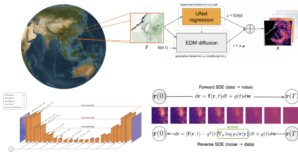
FIGURE 1 – Paradigme deux étages de CORRDIFF (Mardani et al. [15], Fig. 1). Haut : la donnée météorologique LR sert d'abord à prédire la moyenne \mu_{HR} par régression UNet ; cette estimation est ensuite corrigée stochastiquement par un modèle de diffusion EDM produisant le résiduel HR. Bas : SDE directe (data \rightarrow noise) et SDE inverse (noise \rightarrow data) sur lesquelles repose l'échantillonnage du second étage.
