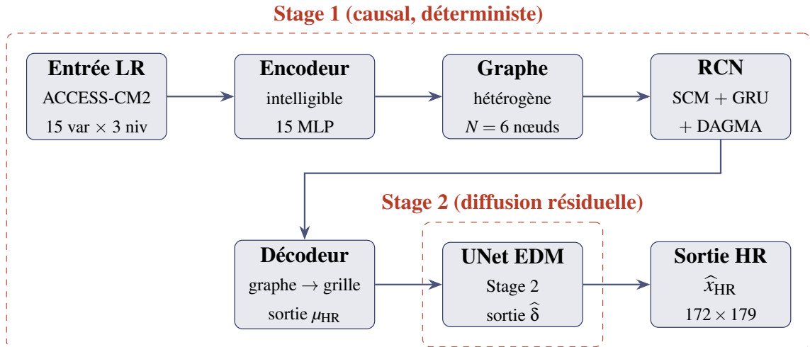
FIGURE 9 – Pipeline architectural d'ORACLE : Stage 1 (causal, déterministe) produit la moyenne \mu_{\text{HR}} par chemin obligatoire à travers le DAG appris ; Stage 2 (diffusion EDM) échantillonne le résiduel \hat{\delta} conditionné par concaténation de canaux.
