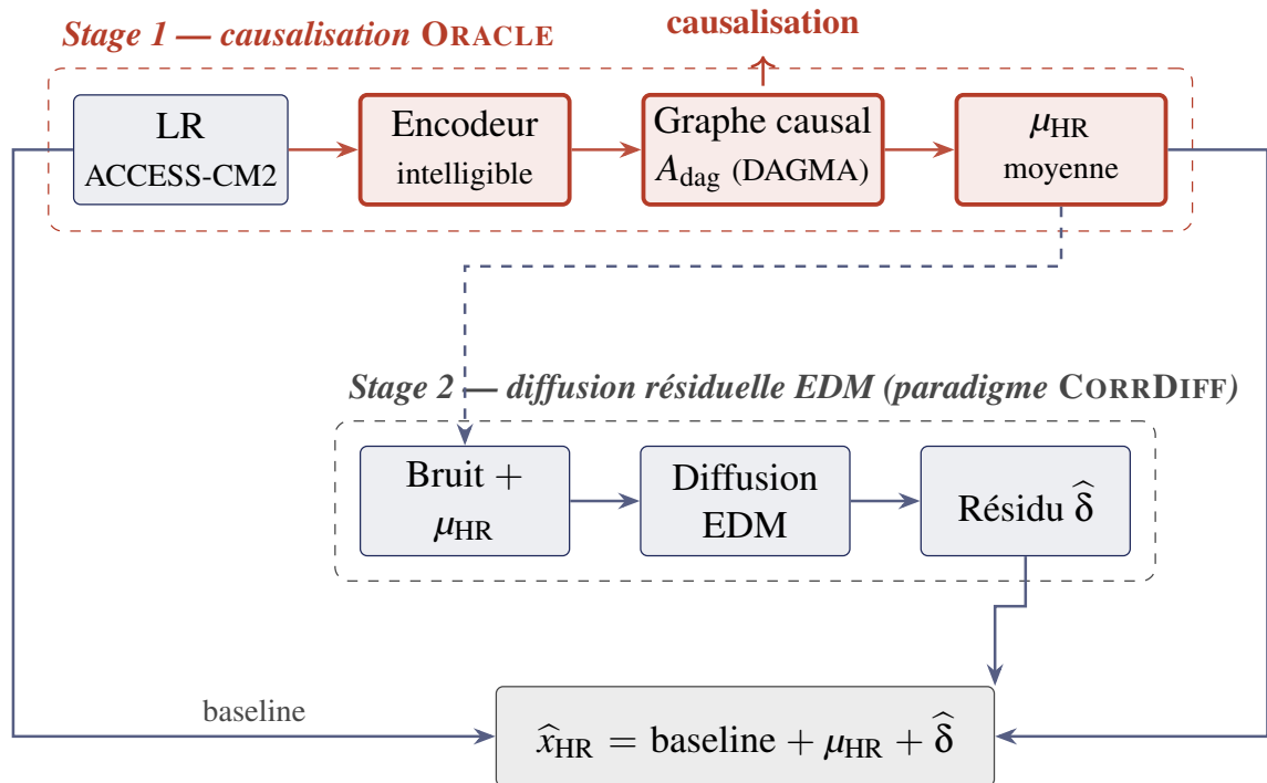
FIGURE 3 – Cartouche conceptuel d’ORACLE : version causalisée du paradigme deux étages de CORRDIFF. L’étage 1 estime \mu_{\text{HR}} via un graphe causal appris ; l’étage 2 échantillonne par diffusion le résiduel \hat{\delta} .
