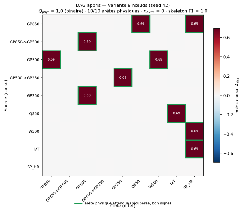
FIGURE 13 – Matrice d'adjacence causale A_{\text{dag}} apprise (variante 9 nœuds, seed 42; ligne = cause, colonne = effet). Les dix arêtes physiquement attendues (encadrées) sont toutes récupérées avec le signe correct, sans arête parasite.
