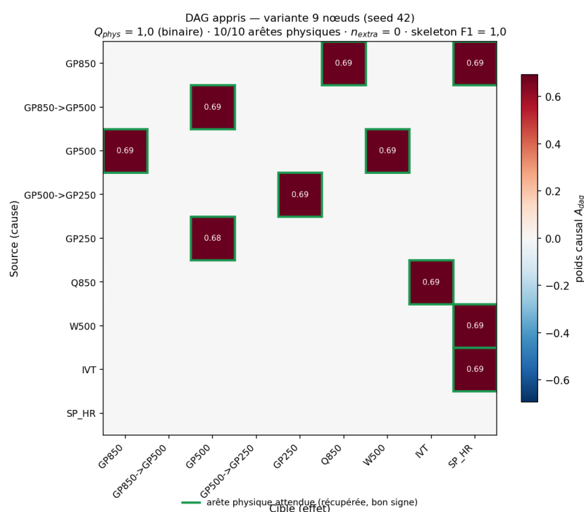
FIGURE 15 – Matrice d’adjacence causale A_{\text{dag}} apprise (variante 9 nœuds, seed 42; ligne = cause, colonne = effet). Les dix arêtes physiquement attendues (encadrées) sont toutes récupérées avec le signe correct, sans arête parasite.
