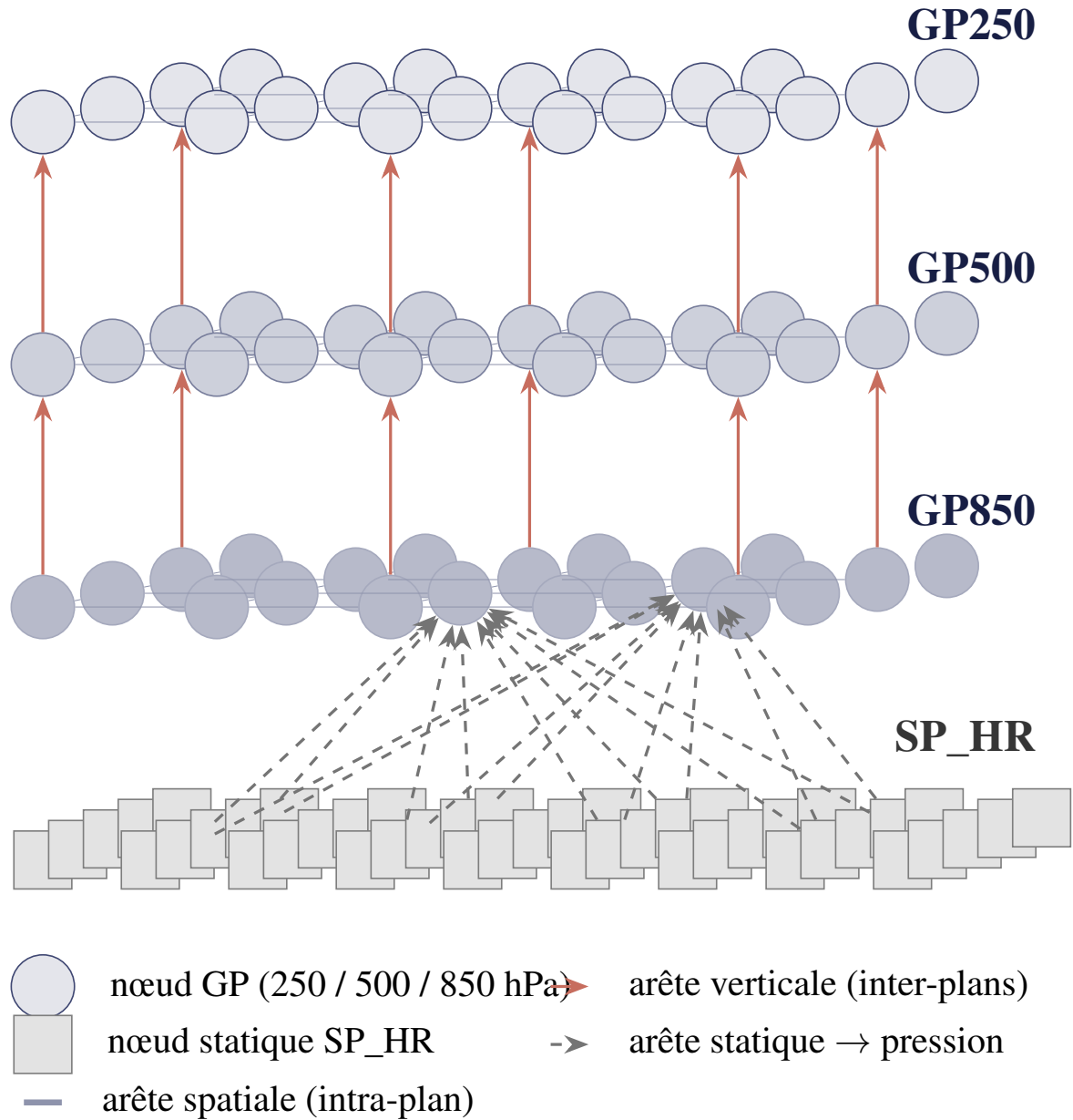
FIGURE 8 – Vue conceptuelle du graphe atmosphérique hétérogène d'ORACLE. Quatre types de nœuds ( GP_{850} , GP_{500} , GP_{250} dynamiques en bleu ; SP_{HR} statique en gris) et trois types d'arêtes (spatiales intra-plan en bleu clair, verticales inter-plans en rouge, statiques-vers-pression en pointillé gris). L'instanciation concrète avec variables nommées et dimensions exactes est différée au chapitre IV.
