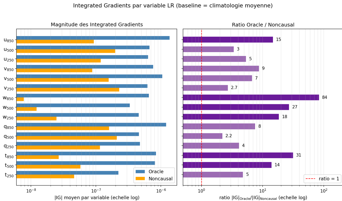
FIGURE 12 – Integrated Gradients (méthode d’attribution mesurant la contribution de chaque variable d’entrée à la prédiction) agrégés par variable LR (u, v, w, q, t sur les niveaux 850, 500, 250 hPa), baseline = climatologie moyenne. Gauche : magnitude moyenne |IG| ; ORACLE (bleu) exploite chaque variable d’un à deux ordres de grandeur plus que la baseline Noncausal (orange). Droite : ratio |IG|_{\text{ORACLE}}/|IG|_{\text{Noncausal}} ; les variables verticales et thermiques ( w_{850}, w_{500}, t_{850} ) ressortent comme leviers principaux.
