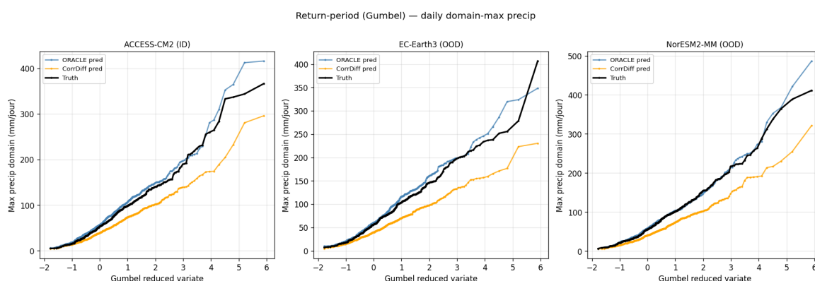
FIGURE 11 – Courbes de période de retour ajustées par la loi de Gumbel, la loi statistique des maxima (la période de retour mesure la rareté d'un événement : un événement « centennal » ne survient en moyenne qu'une fois par siècle) pour la précipitation journalière maximale sur le domaine, en distribution (ACCESS-CM2) et hors distribution (EC-Earth3, NorESM2-MM). ORACLE (bleu) suit la vérité (noir) jusqu'aux périodes de retour les plus longues sur les trois GCM; la baseline Noncausal (orange) sature systématiquement en dessous des extrêmes observés.
