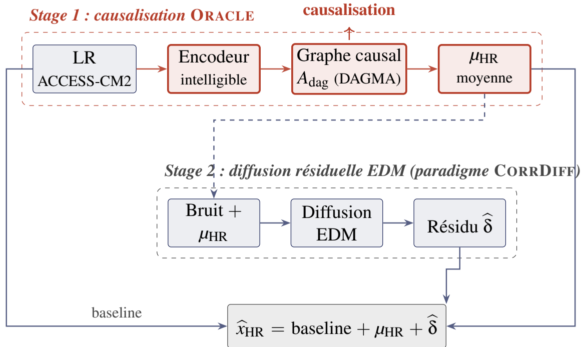
FIGURE 3 – Cartouche conceptuel d'ORACLE : version causalisée du paradigme deux étages de CORRDIFF. L'étage 1 estime \mu_{HR} via un graphe causal appris ; l'étage 2 échantillonne par diffusion le résiduel \delta .
