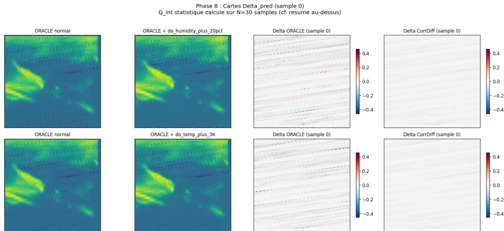
FIGURE 13 – Cartes des perturbations contrôlées \Delta q + 20\% et \Delta t + 3\text{ K} . Signes physiques cohérents avec la relation de Clausius-Clapeyron sur les deux perturbations testées. Les amplitudes, de l'ordre de 10^{-3} en unités relatives, rendent les cartes visuellement peu contrastées : les statistiques quantitatives (moyennes et IC bootstrap) figurent au Tableau X.
