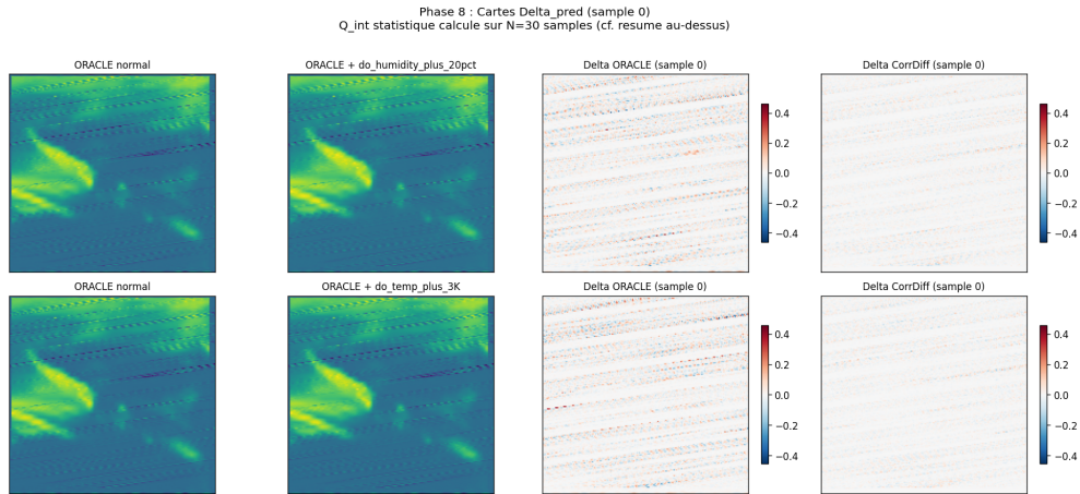
Figure 2 — Cartes des perturbations contrôlées \Delta q + 20\% et \Delta t + 3 K. Signes physiques cohérents avec la relation de Clausius-Clapeyron sur les deux perturbations testées.
