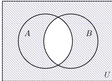
Figure 8: Visualización de la propiedad \sim (A \cap B) = \sim A \cup \sim B .
