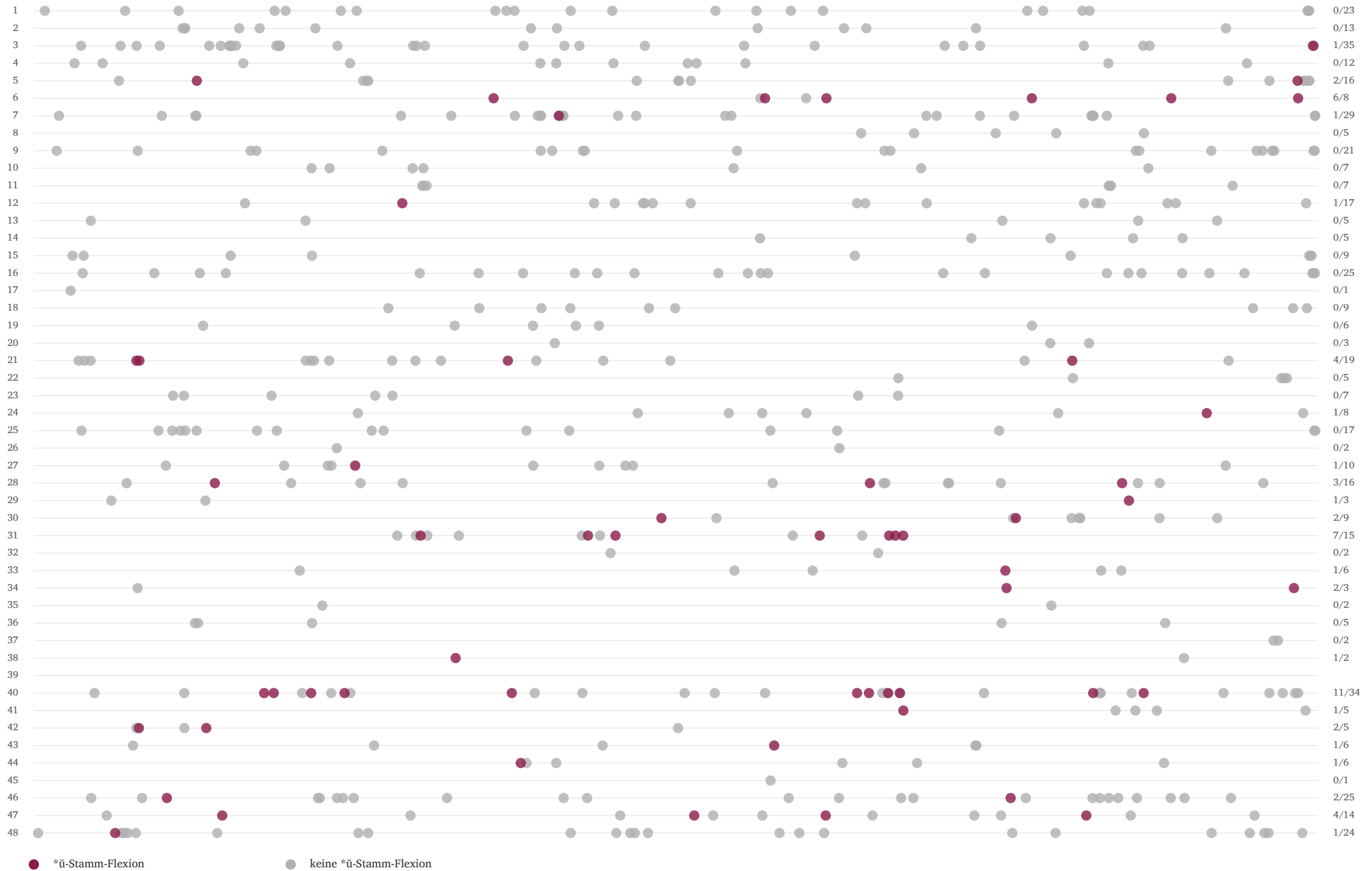
DtSg — *ŭ-Stamm-Flexion vs. andere Flexion
