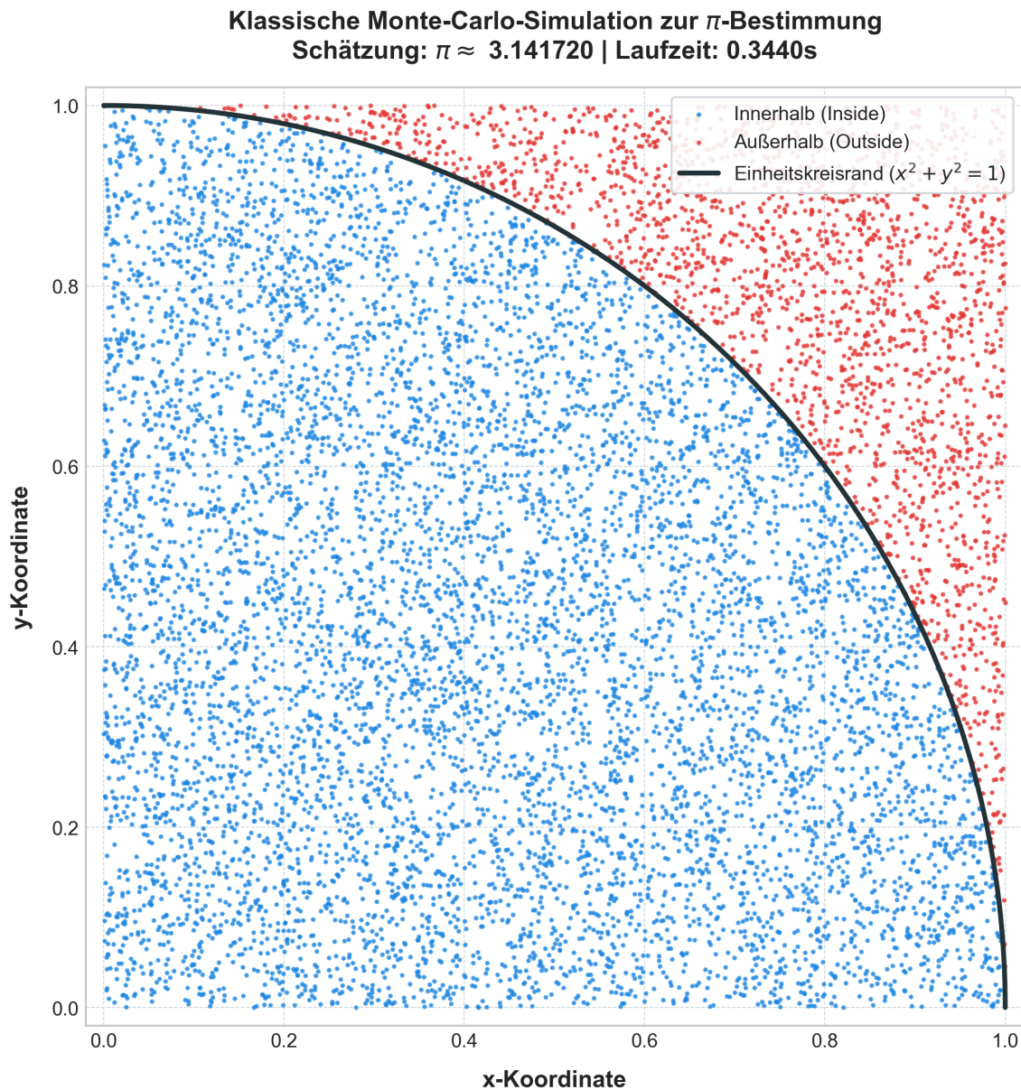
Figure 4: Geometrischer Pi-Schätzungs-Scatterplot
