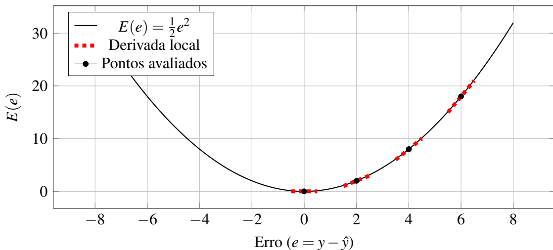
Figura 4 – Função de erro quadrático e segmentos de retas tangentes representando a derivada em diferentes pontos.
