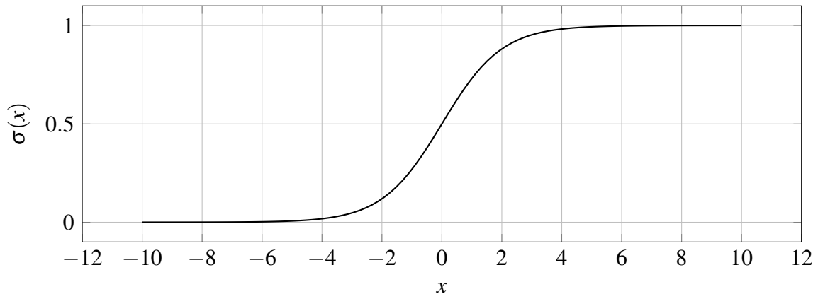
Figura 2 – Função Sigmoide
