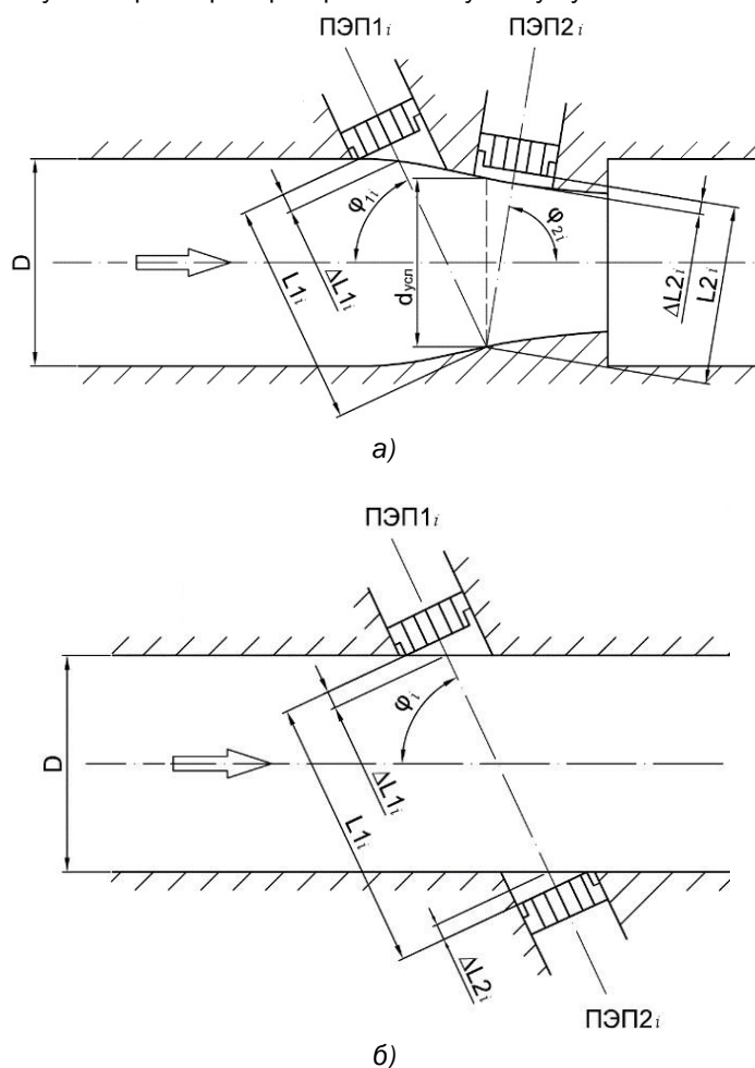
Рисунок А.1 – Измерительные схемы ИРВИС-Ультра-ПП а) – V-образная с каналом специальной формы; б) – диагональная
