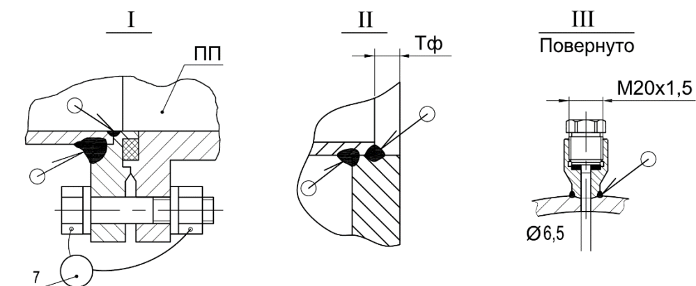
Рисунок Г.3 – Составные части участка «врезки» ИРВИС-Ультра-Пп DN80-400
