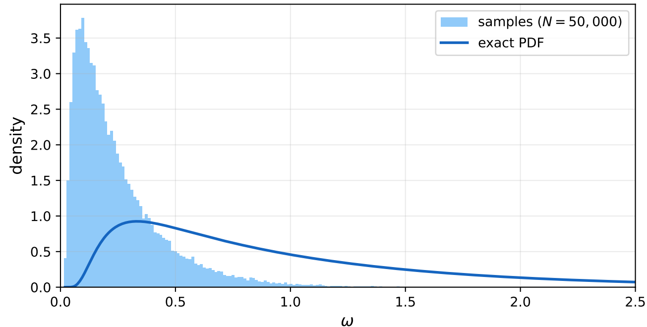
Pólya-Gamma distribution PG(1, 0)
