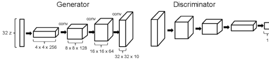
Figura 2.3: Representação da arquitetura da GAN utilizada no paper. Fonte: (Volz et al., 2018)
