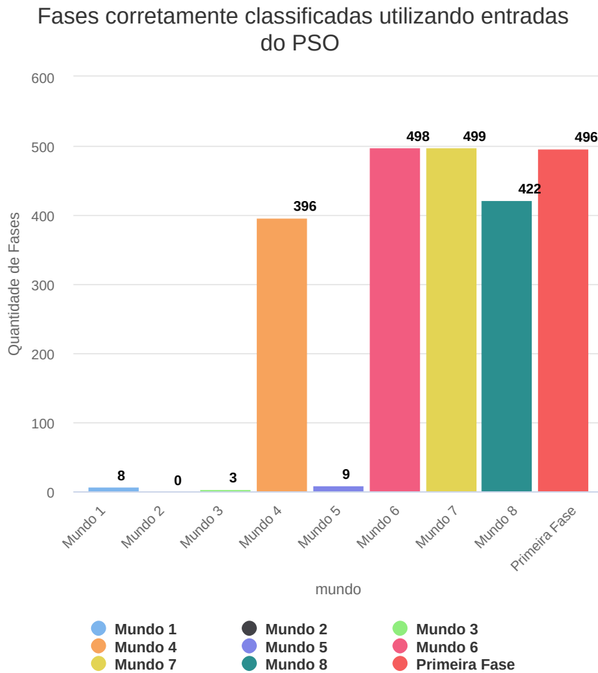
Figura 5.15: Classificação correta das entradas do PSO
