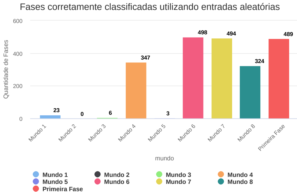
Figura 5.13: Classificação corretas das entradas aleatórias
