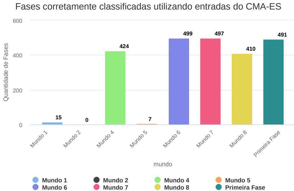
Figura 5.14: Classificação corretas das entradas do CMA-ES
