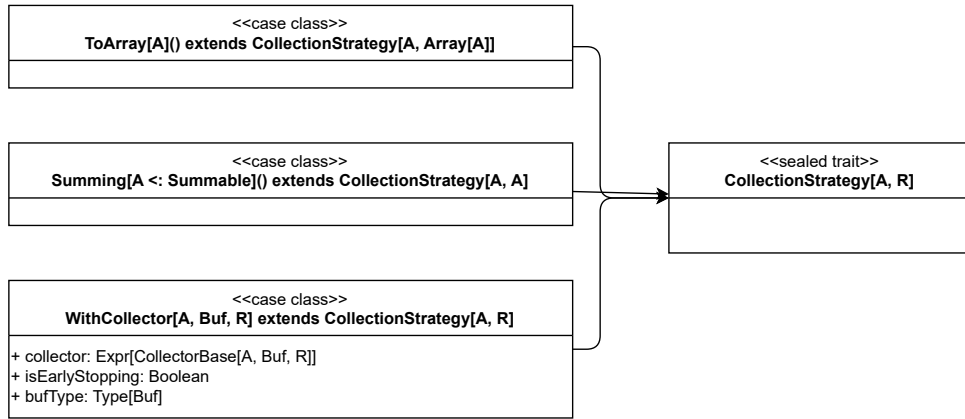
Figura 5.5: Diagramma UML delle classi per la gerarchia CollectionStrategy[A, R] . Summable è definito come union type dei tipi numerici Int , Long , Float e Double .
