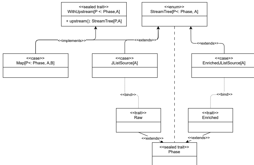
Figura 5.3: Struttura semplificata della Stream IR. La relazione non standard «bind», indica la specializzazione di un parametro di tipo mediante un tipo concreto. nel diagramma, il parametro di fase P viene specializzato con Raw o Enriched .
