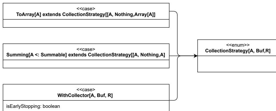
Figura 5.5: Diagramma UML delle classi per la gerarchia CollectionStrategy . Summable è definito come union type dei tipi numerici Int , Long , Float e Double .
