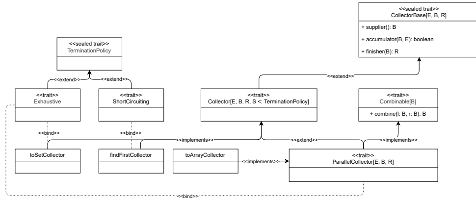
Figura 5.2: Gerarchia dei Collector e relative politiche di terminazione. La non standard relazione «bind», rappresenta la specializzazione di un parametro di tipo con un tipo concreto. in questo caso, il parametro S con una specifica TerminationPolicy .
