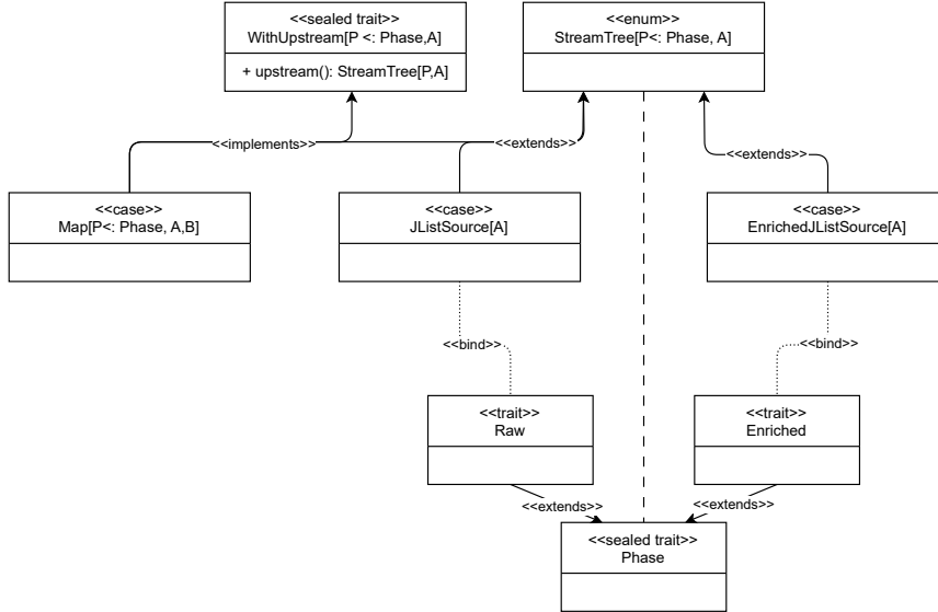
Figura 5.3: Struttura semplificata della Stream IR. La relazione non standard «bind» indica la specializzazione di un parametro di tipo mediante un tipo concreto. Nel diagramma, il parametro di fase P viene specializzato con Raw o Enriched.
