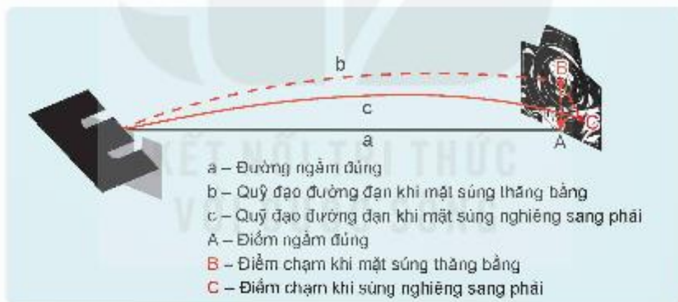
Hình 6.6. Ảnh hưởng của mặt súng không thẳng bằng
