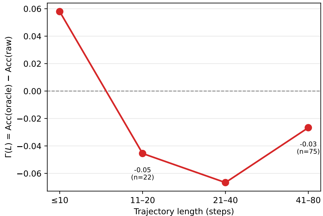
Context gap \Gamma(L)
