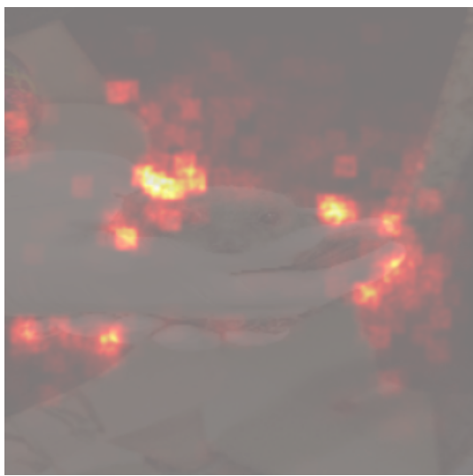
Smoothed Gradients
