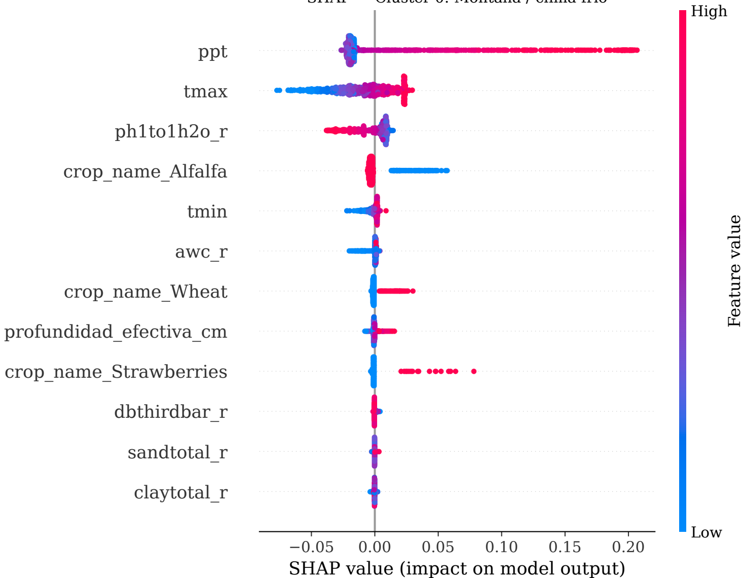
SHAP — Cluster 0: Montaña / clima frío
