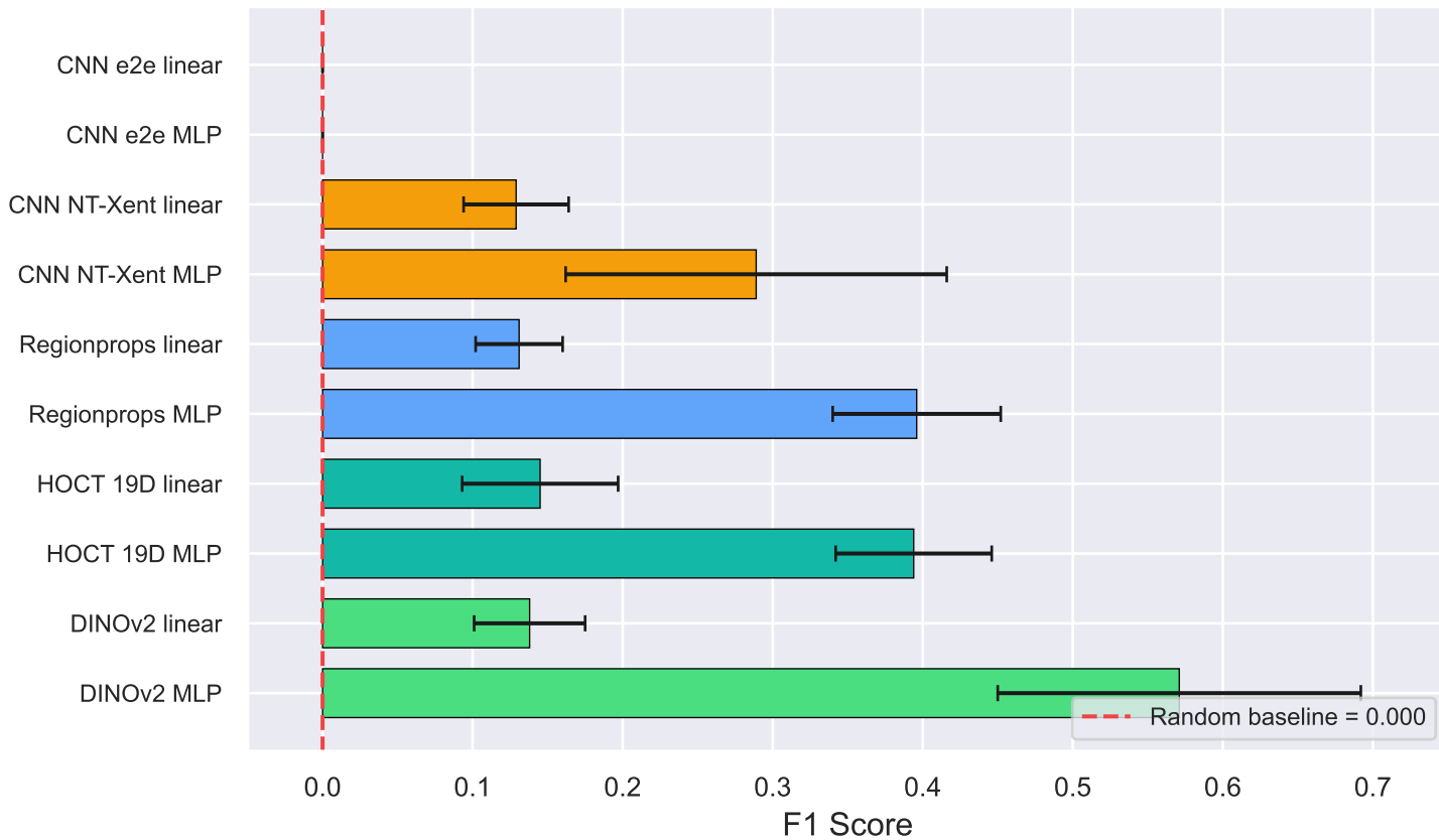
Edge Prediction — F1 Score (5-fold CV)
