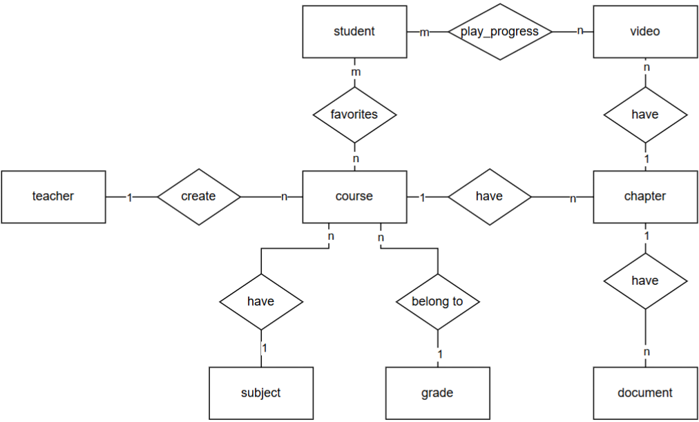
课程管理 ER 图
