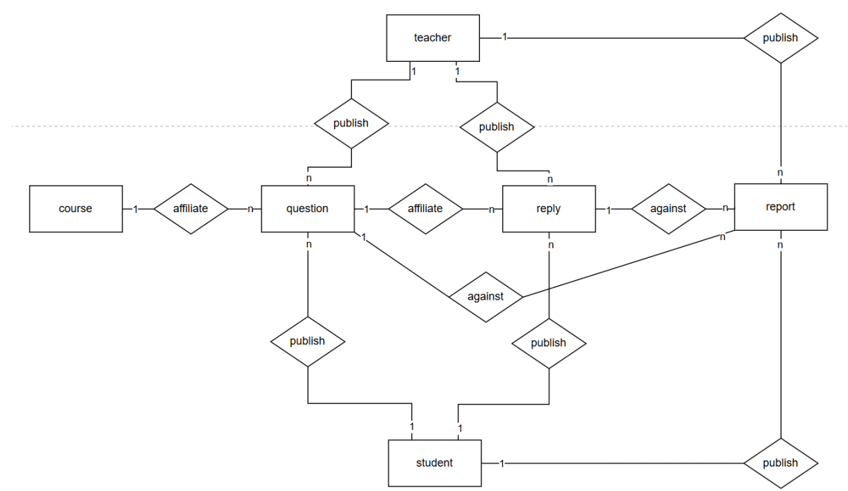
评论系统 ER 图
