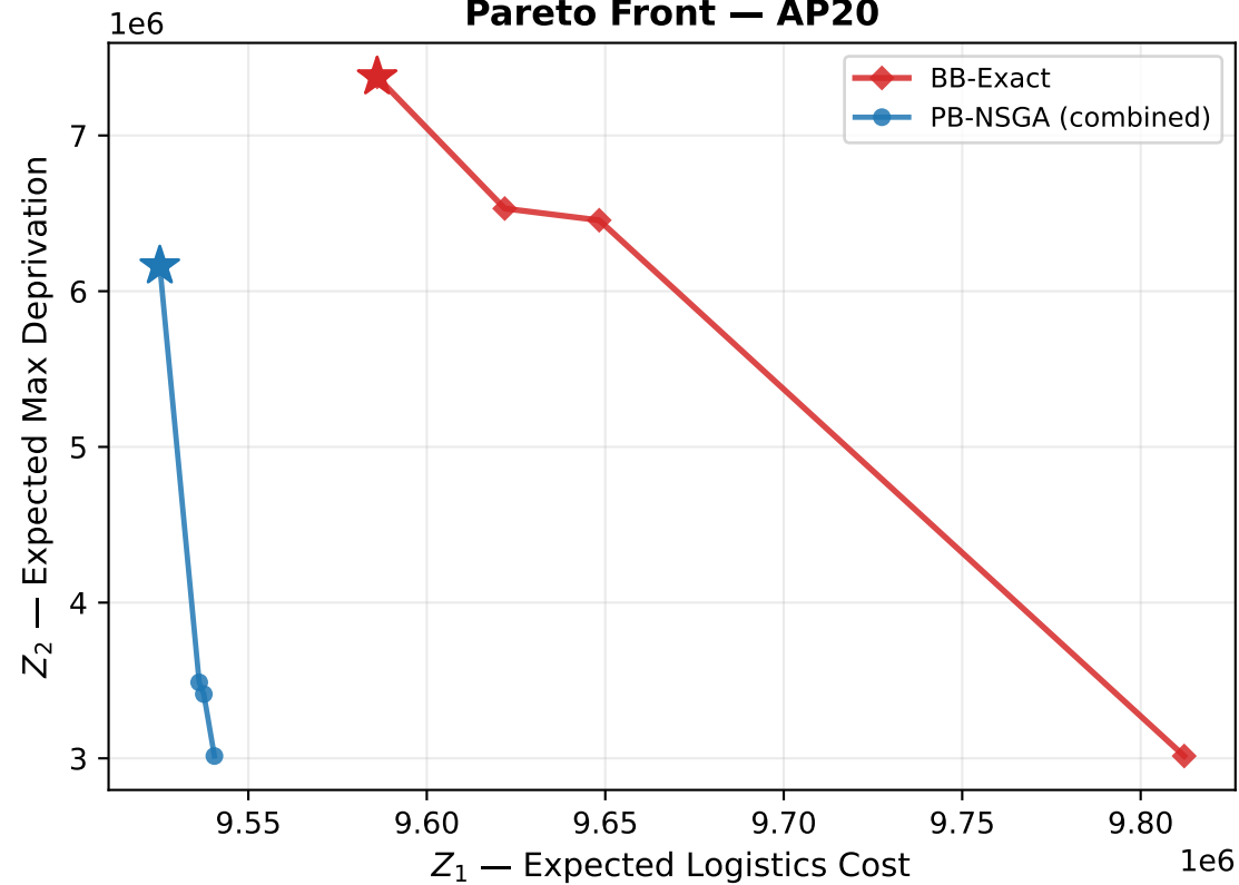
Pareto Front — AP20
