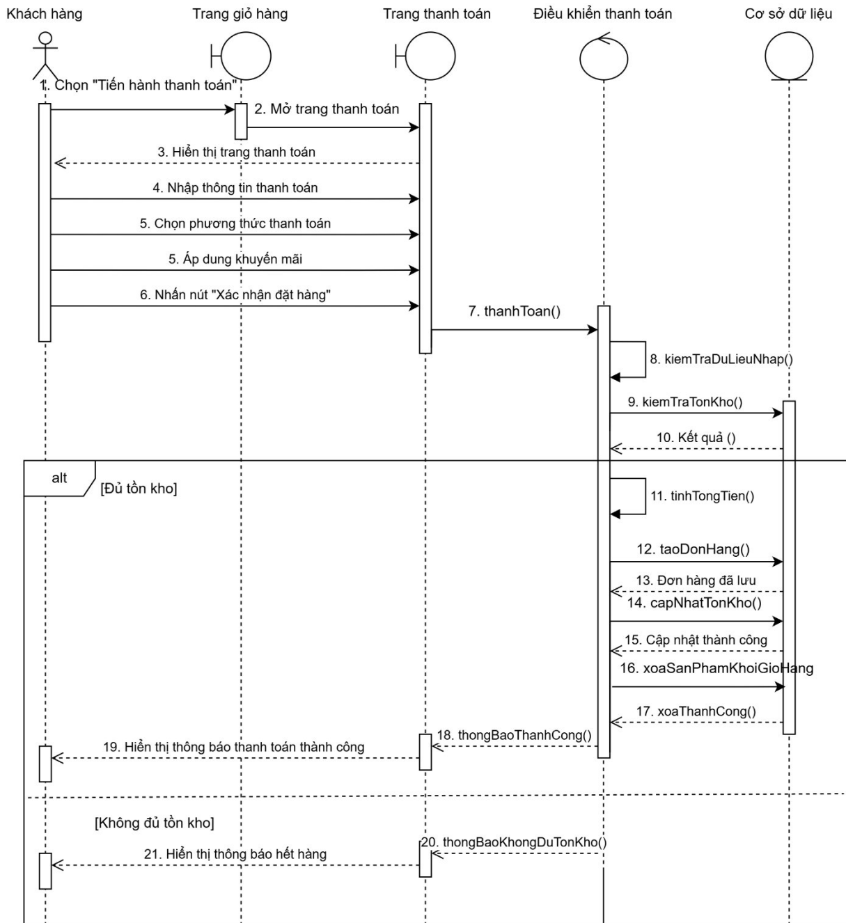
Hình 4-3 Sequence Diagram – Thanh toán
