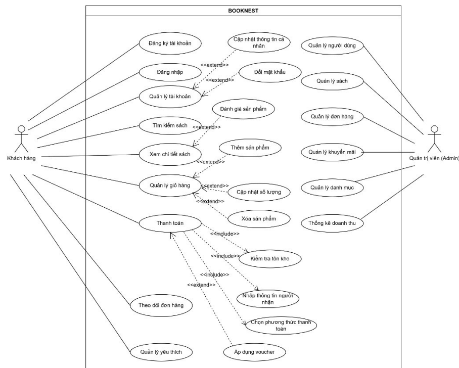
Hình 4-1 Use Case Diagram
