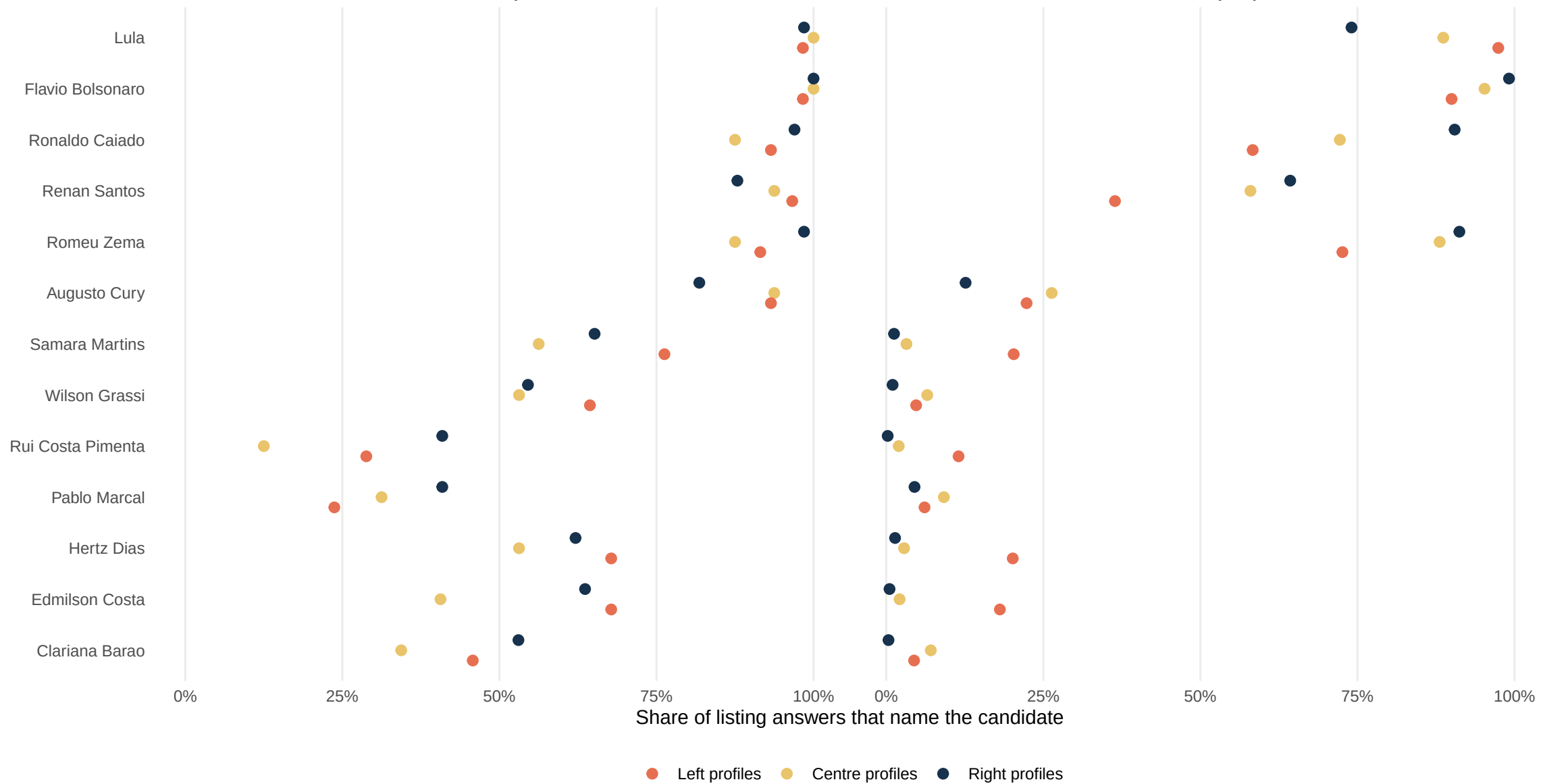
Claude Opus 5
