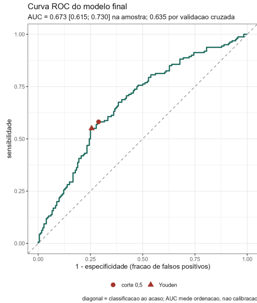
Figura 18: Curva ROC do modelo final. Os pontos marcam o corte de 0,5 e o de Youden (0,52); a diagonal corresponde à classificação ao acaso.
