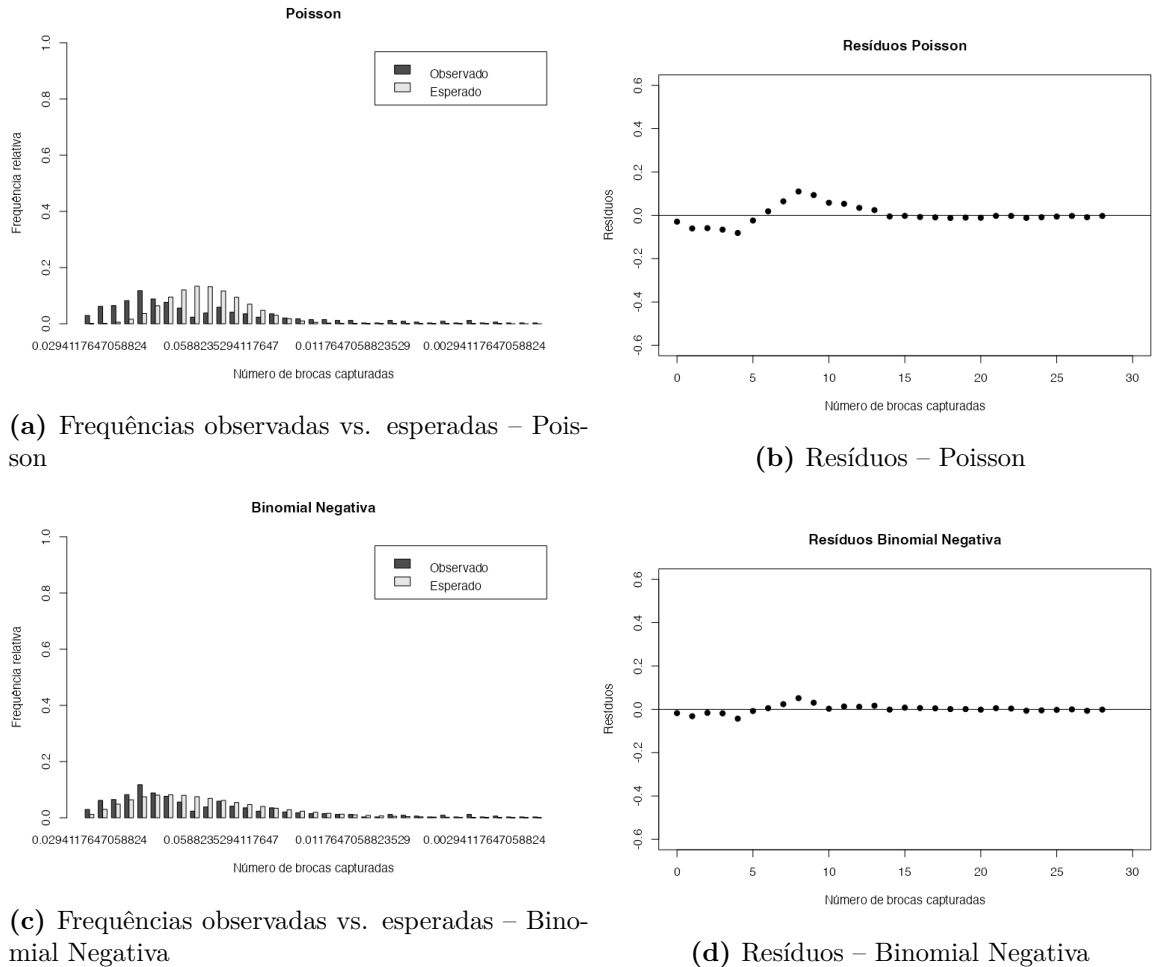
Figura 13: Comparação entre as frequências relativas observadas e esperadas do número de brocas capturadas, e respectivos resíduos, sob os modelos Poisson e Binomial Negativa.
