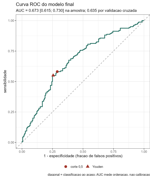
Figura 17: Curva ROC do modelo final. Os pontos marcam o corte de 0,5 e o de Youden (0,52); a diagonal corresponde à classificação ao acaso.
