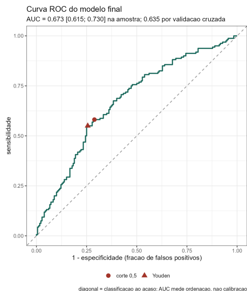
Figura 14: Curva ROC do modelo final. Os pontos marcam o corte de 0,5 e o de Youden (0,52); a diagonal corresponde à classificação ao acaso.
