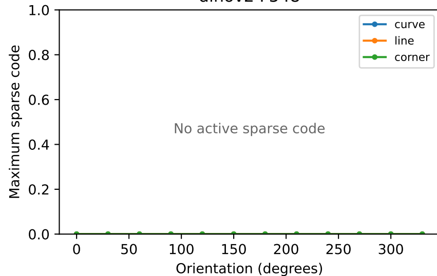
dinov2 F548
