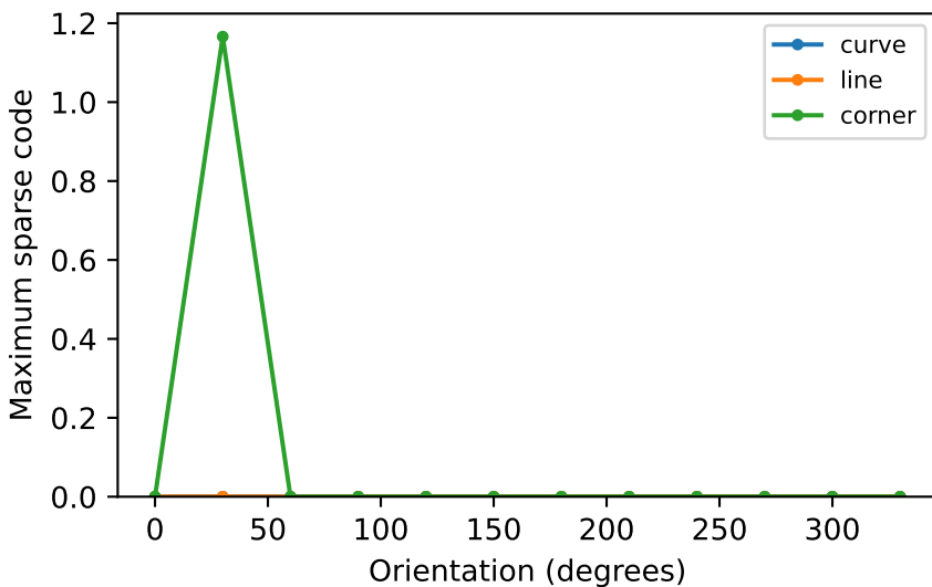
dinov2 F760
