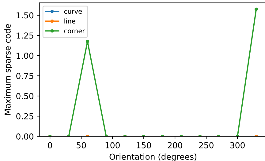
dinov2 F548
