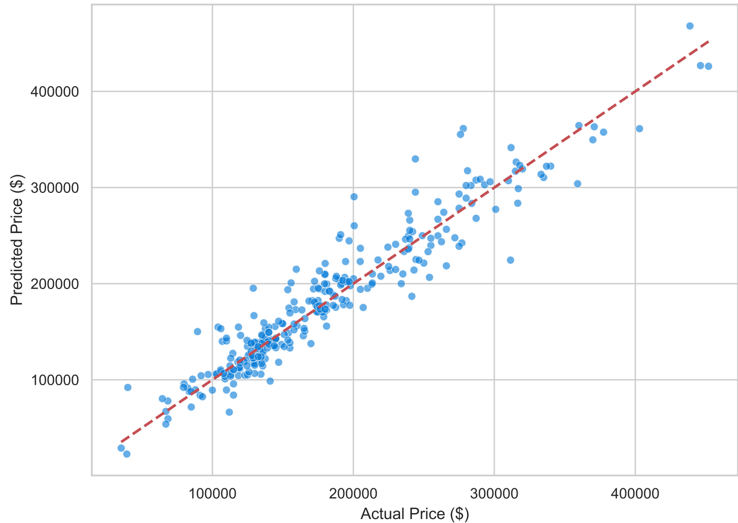
Actual vs. Predicted Prices
