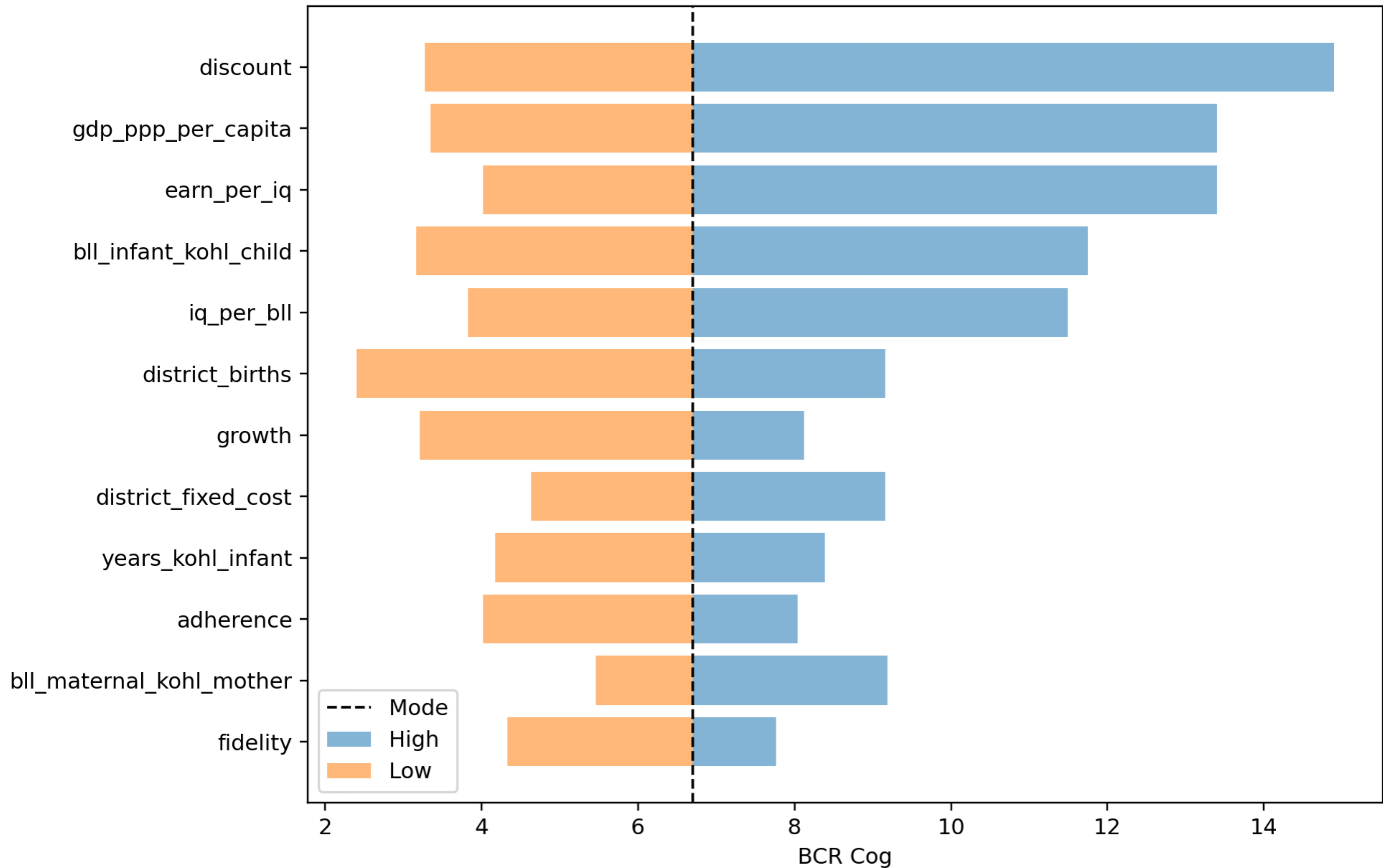
Tornado Diagram: Kohl BCR Cog
