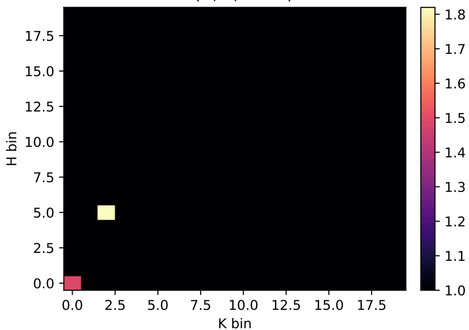
T^*(H, K, k=10)
