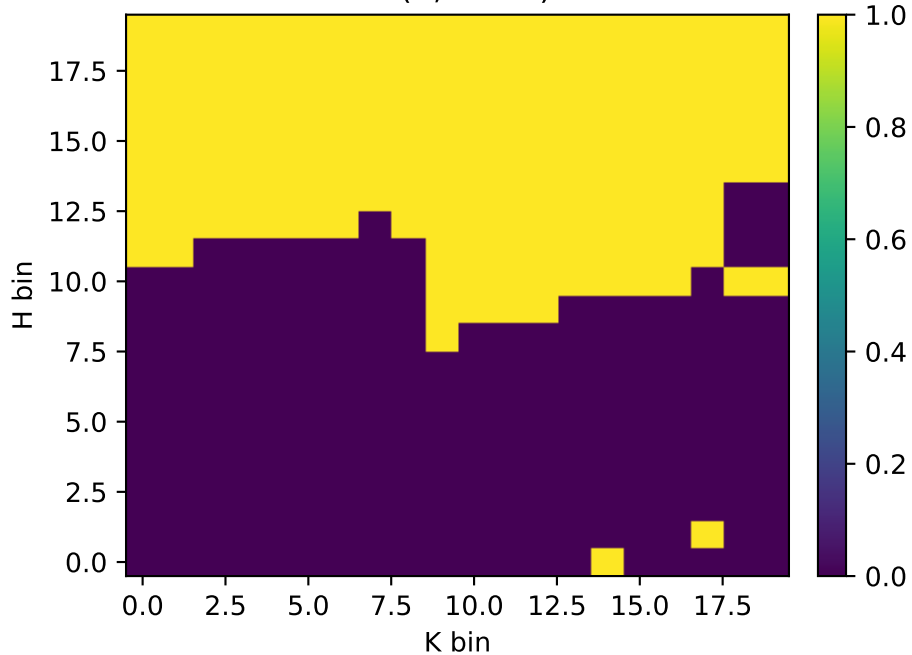
h^*(K, k=14)
