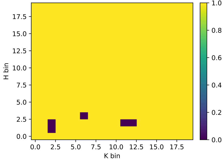
h^*(K, k=6)
