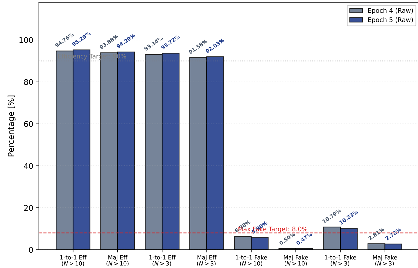
(d) Benchmark Progression: Epoch 4 vs Epoch 5 (genStatus \in [0, 1] )
