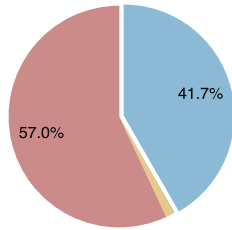
Qwen3-VL-235B-A22B
