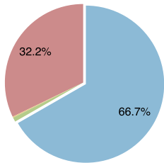
GPT-5.4-mini
