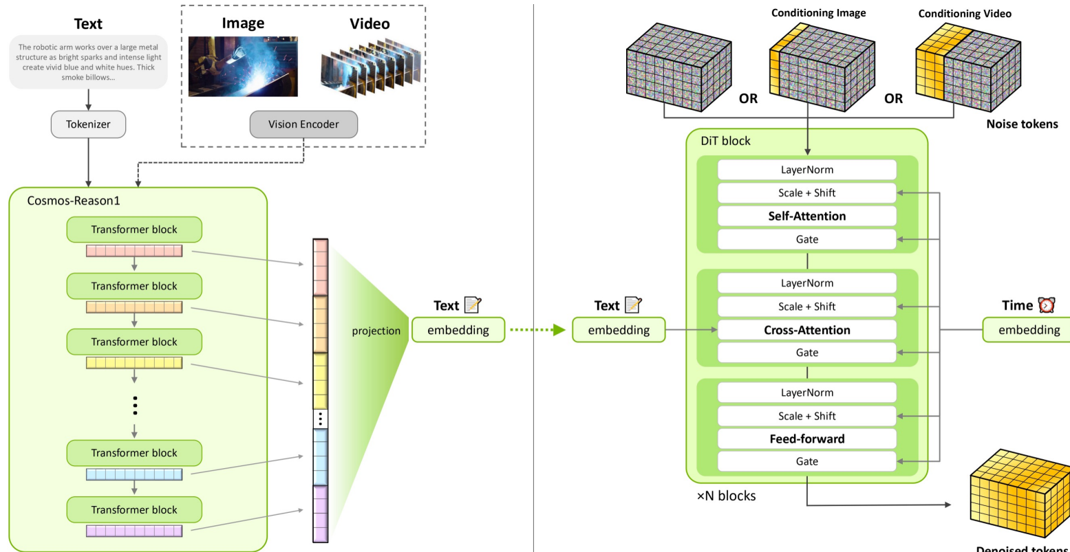
Cosmos-Predict2.5 공식 아키텍처 (NVIDIA 테크리포트)
