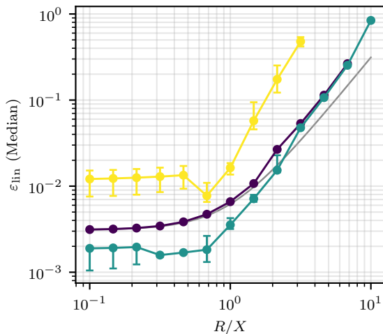
(d) const_x: Linearisierungsfehler
